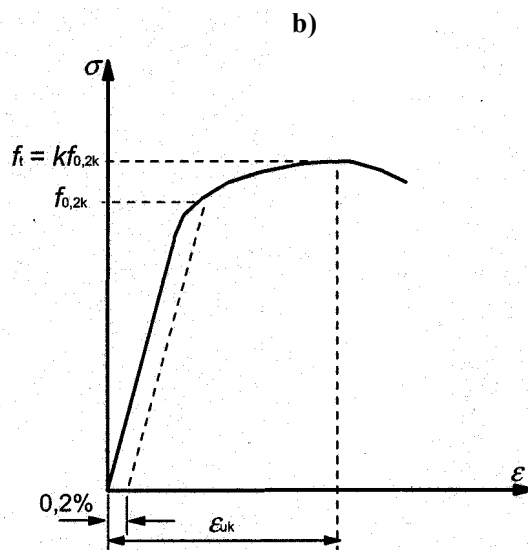
b) ocel za studena tvářená zvyšuje se mez kluzu a pevnosti, zmenšuje tažnost
